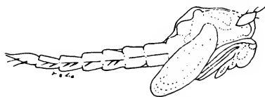
Fig. 562. Tanypus illinoensis Mall.
